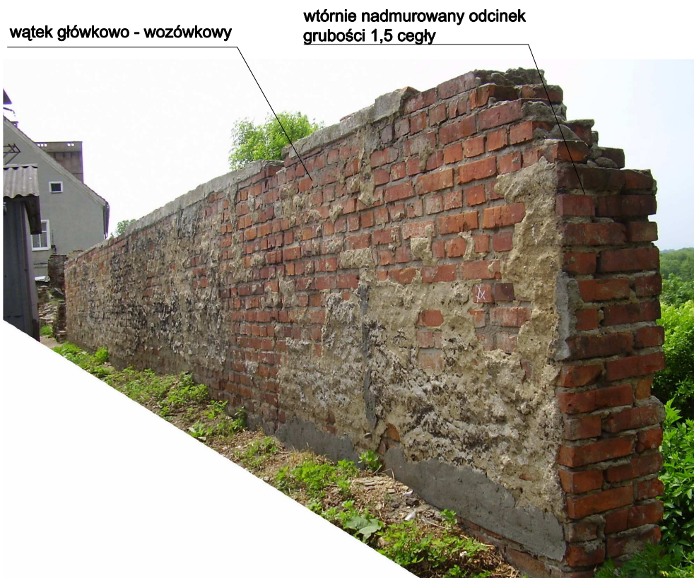
fot. 31 Biała - odcinek miejskich murów obronnych przy ul. Szkolnej Północny odcinek muru - wewnętrzne lico muru z cegły mechanicznej
