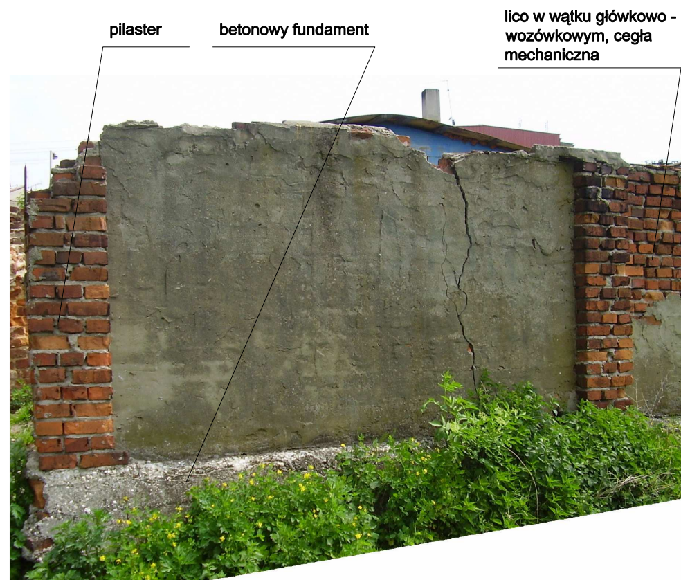
fot. 32 Biała - odcinek miejskich murów obronnych przy ul. Szkolnej Północny odcinek muru, fragment lica zewnętrznego - widok od zachodu
