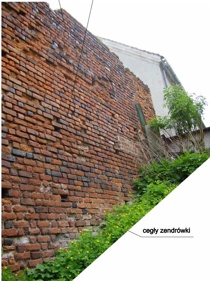
fot. 16 Biała - odcinek miejskich murów obronnych przy ul. Szkolnej Zewnętrzne lico muru - część południowa
