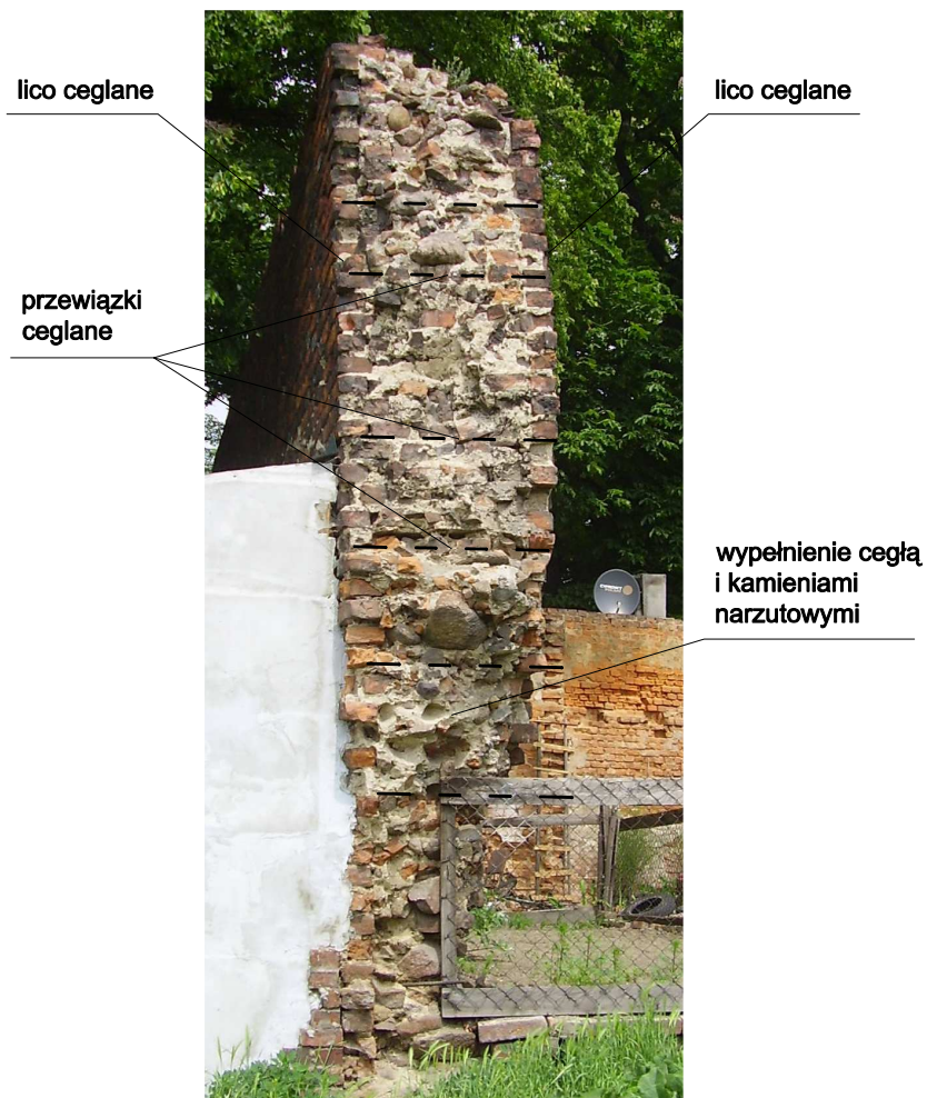
fot. 7 Miejskie mury obronne w Białej Mur obronny na północ od odcinka badanego - przekrój
